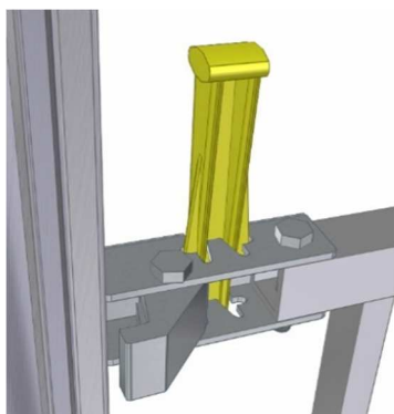
Öppen tving
